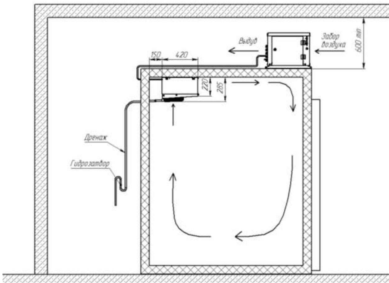
Рис.4 Вариант расположения агрегата на камере.
