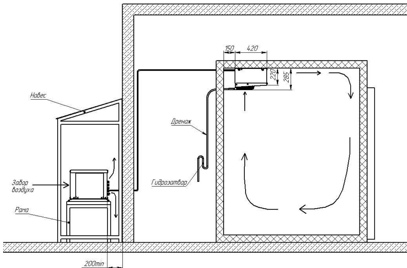
Рис.5 Вариант расположения агрегата на раме (уличный вариант). (Рекомендуется располагать под навесом).
