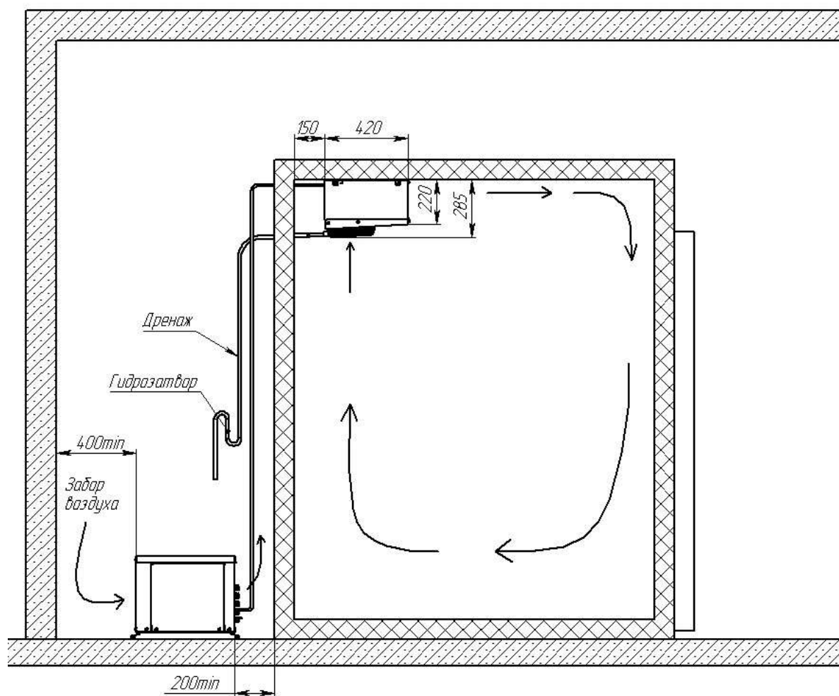
Рис.4 Вариант расположения агрегата на камере.
